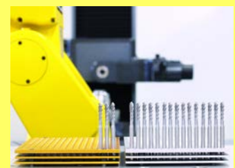
Automatische Sortierung fehler- hafter und korrekter Werkzeuge
